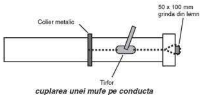
Fig. 6 Îmbinare conducte
