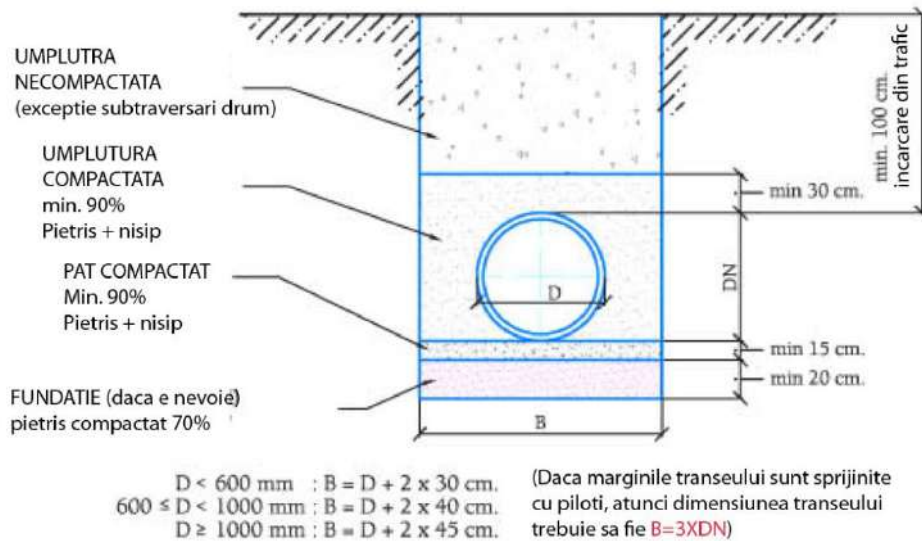
Fig. 2 Profil transversal
