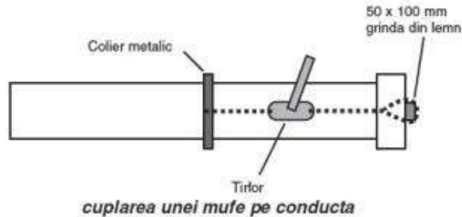
Fig. 9 Îmbinare conducte
