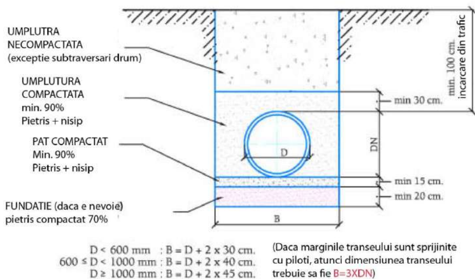
Fig. 5 Profil transversal
